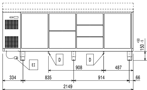
Boční
